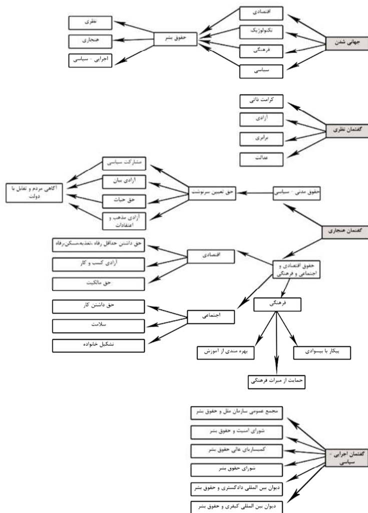
شکل ۱: الگوی پژوهش
